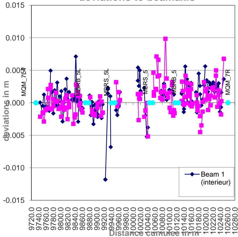
LSS 4 - chambres à vide - radial deviations to beamaxis
